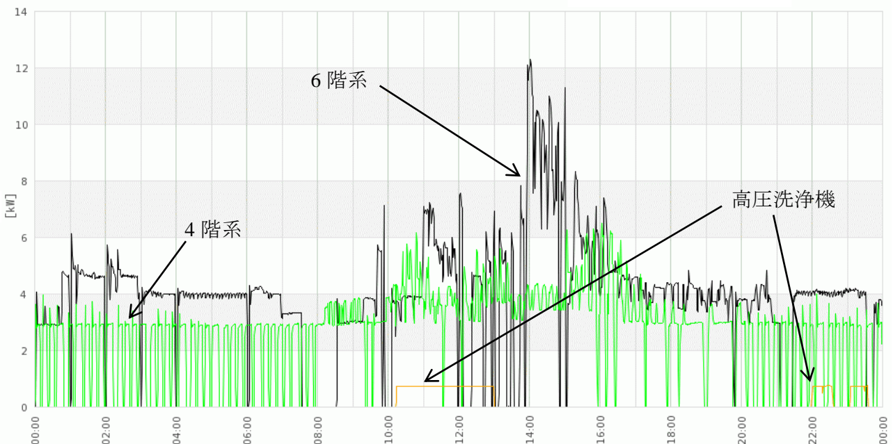
図5 2015/08/25 のエアコン室外機と高圧洗浄機の使用電力データ
