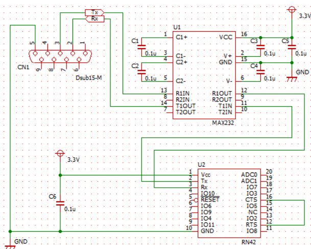
図4 Bluetoothアダプタ設定回路
